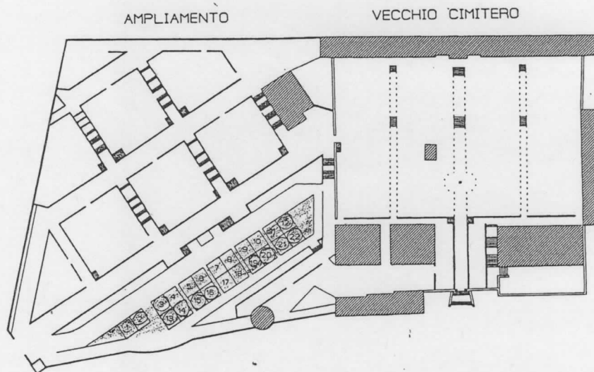
PLANIMETRIA GENERALE SCALA 1:1000
